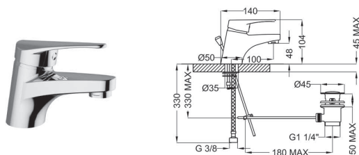
ΜΠΑΤΑΡΙΑ ΝΙΠΤΗΡΑ με μακρύ ρουξούνι και αυτόματη βαλβίδα
