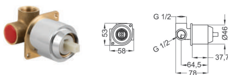
ΕΝΤΟΙΧΙΖΟΜΕΝΟΣ ΜΗΧΑΝΙΣΜΟΣ ΜΠΑΤΑΡΙΑΣ μίας εξόδου νιπτήρα
