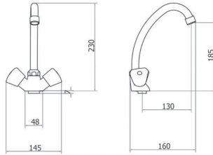
ΜΠΑΤΑΡΙΑ ΜΙΑΣ ΟΠΗΣ 14 cm ρουξούνι
