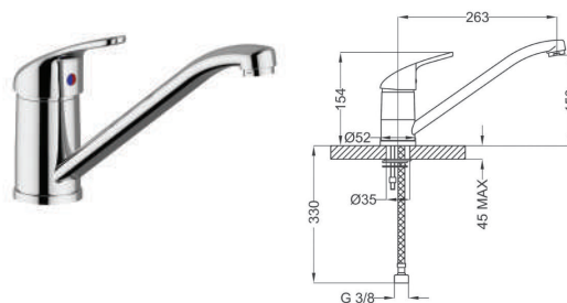
ΜΠΑΤΑΡΙΑ ΝΕΡΟΧΥΤΗ ΠΑΓΚΟΥ ΠΛΑΓΙΑ
