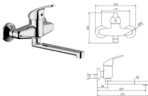
ΜΠΑΤΑΡΙΑ ΝΕΡΟΧΥΤΗ ΠΑΓΚΟΥ ΤΟΙΧΟΥ
