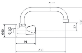
ΜΠΑΤΑΡΙΑ ΜΟΝΗ περιστρεφόμενη τοίχου
