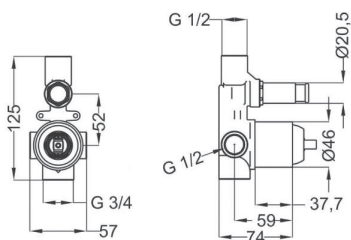
ΕΝΤΟΙΧΙΖΟΜΕΝΟΣ ΜΗΧΑΝΙΣΜΟΣ ΜΠΑΤΑΡΙΑΣ δύο ροών
