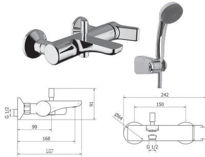
ΜΠΑΤΑΡΙΑ ΜΠΑΝΙΟΥ αναμεικτική με ντουζ
