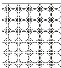
ΠΛΑΚΑ ΜΕ ΚΟΜΒΟΥΣ ΠΑΧΟΥΣ 15mm με βήμα 10 cm
