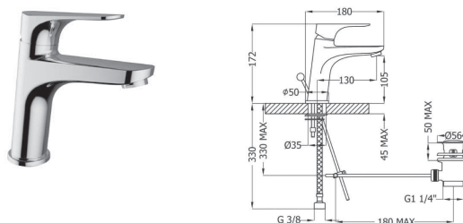
ΜΠΑΤΑΡΙΑ ΝΙΠΤΗΡΑ με αυτόματη βαλβίδα
