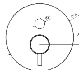
ΛΑΒΗ - ΡΟΖΕΤΑ - ΔΙΑΝΕΜΗΤΗΣ για ντουζ εντοιχισμού /Μαύρη
