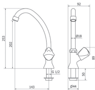
ΜΠΑΤΑΡΙΑ ΜΟΝΗ περιστρεφόμενη πάγκου
