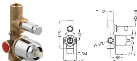
ΕΝΤΟΙΧΙΖΟΜΕΝΟΣ ΜΗΧΑΝΙΣΜΟΣ ΜΠΑΤΑΡΙΑΣ δύο εξόδων ντουζ
