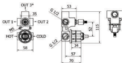
ΕΝΤΟΙΧΙΖΟΜΕΝΟΣ ΜΗΧΑΝΙΣΜΟΣ ΜΠΑΤΑΡΙΑΣ με περιστροφικό διανεμητή δύο ροών
