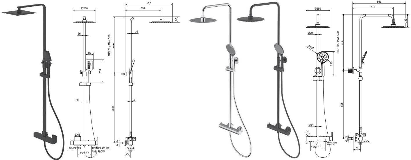
ΣΤΗΛΗ ΝΤΟΥΖ ΤΕΤΡΑΓΩΝΗ με σπιδράλ τηλέφωνο και μπαταρία
