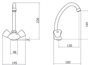
ΜΠΑΤΑΡΙΑ ΜΙΑΣ ΟΠΗΣ 20 cm ρουξούνι
