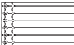
ΠΛΑΚΑ ΜΕ ΕΓΚΟΠΕΣ ΠΑΧΟΥΣ 15mm με βήμα 10 cm
