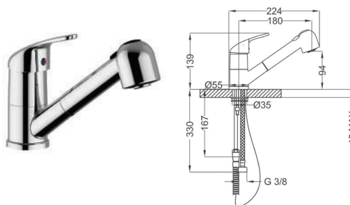
ΜΠΑΤΑΡΙΑ ΝΕΡΟΧΥΤΗ ΠΑΓΚΟΥ με σπирάλ και ντουζ
