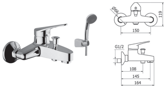
ΜΠΑΤΑΡΙΑ ΜΠΑΝΙΟΥ αναμεικτική με ντουζ
