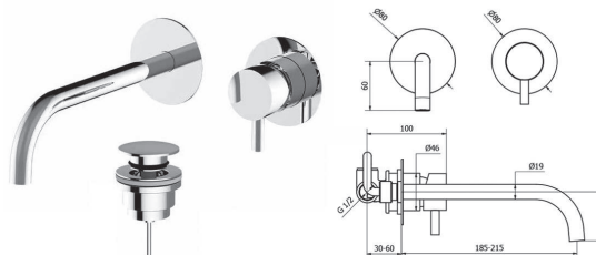
ΡΟΥΞΟΥΝΙ-ΛΑΒΗ-ΡΟΖΕΤΑ ΝΙΠΗΤΡΑ ΑΝΑΜΕΙΚΤΙΚΗ ΕΝΤΟΙΧΙΣΜΟΥ χωρίς βαλβίδα / χρωμέ
